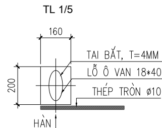
TAI BẮT TIẾP ĐỊA
