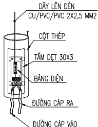
CHI TIẾT BẢNG ĐIỆN
