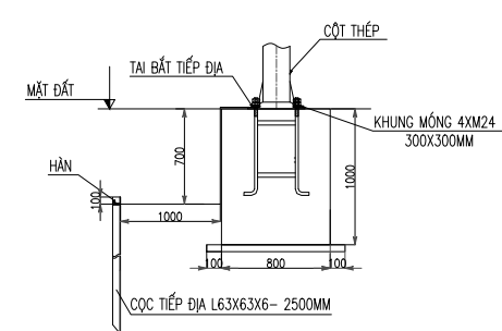
TIẾP ĐỊA CHO CỘT ĐÈN
