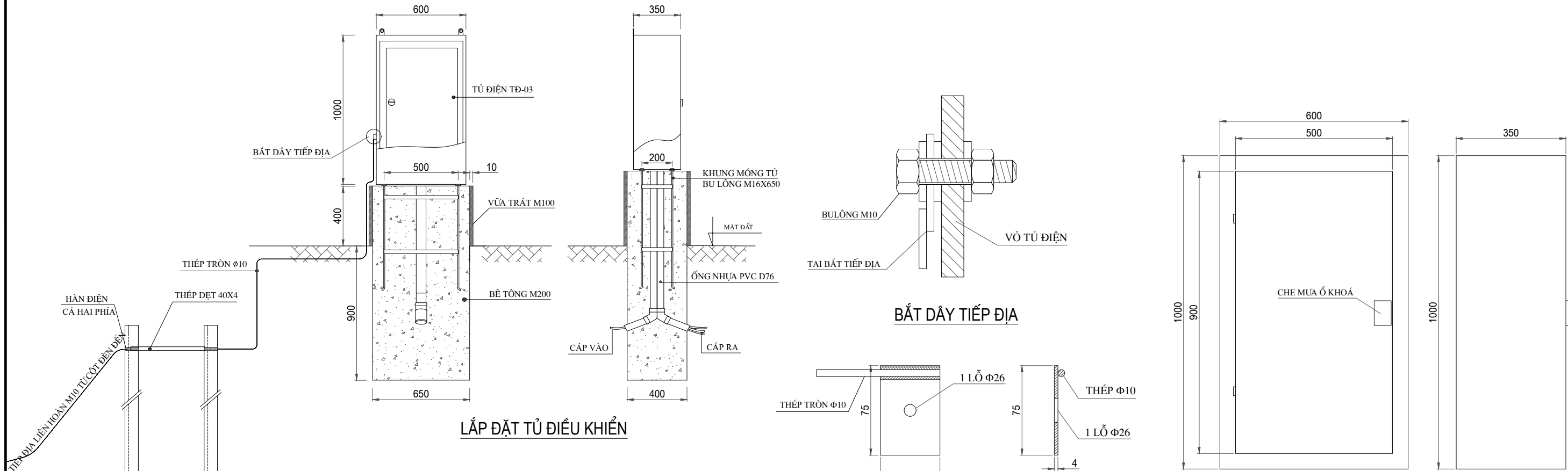
VỎ TỦ ĐIỆN
