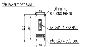
CHI TIẾT BẢNG ĐIỆN
