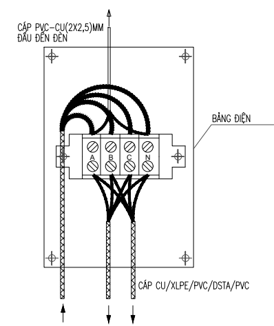
PHƯƠNG THỨC ĐẦU NỐI TẠI CỘT RỄ NHÁNH
