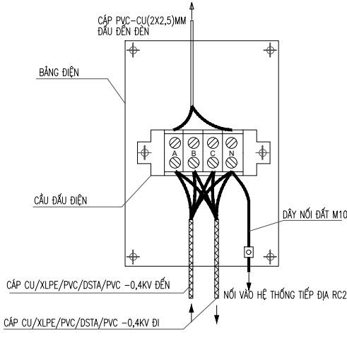
PHƯƠNG THỨC ĐẦU NỐI TẠI CỘT
