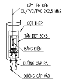
CHI TIẾT BẢNG ĐIỆN
