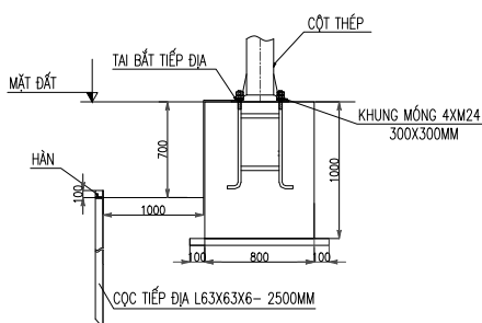
TIẾP ĐỊA CHO CỘT ĐÈN
