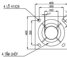
KHUNG MÓNG CỘT ĐÈN CHIẾU SÁNG 4XM24-300X300MM
