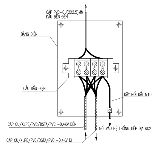
PHƯƠNG THỨC ĐẦU NỐI TẠI CỘT
