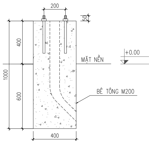
TAI BẮT TIẾP ĐỊA
