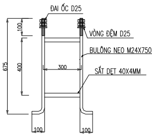
KHUNG MÓNG CỘT ĐÈN CHIẾU SÁNG 4XM24-300X300MM
