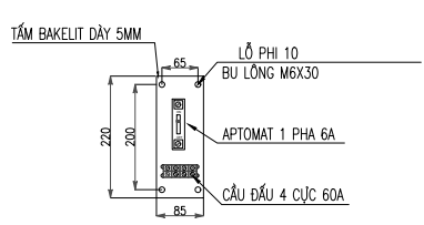
CHI TIẾT BẢNG ĐIỆN
