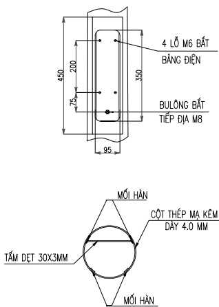
MÓNG CỘT ĐÈN CHIẾU SÁNG - CỘT 8M
