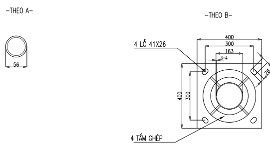
KHUNG MÓNG CỘT ĐÈN CHIẾU SÁNG
