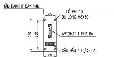
CHI TIẾT BẢNG ĐIỆN
