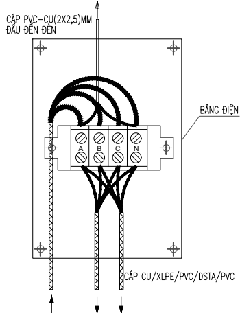
PHƯƠNG THỨC ĐẦU NỐI TẠI CỘT RỄ NHÁNH
