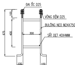
KHUNG MÓNG CỘT ĐÈN CHIẾU SÁNG 4XM24-300X300MM
