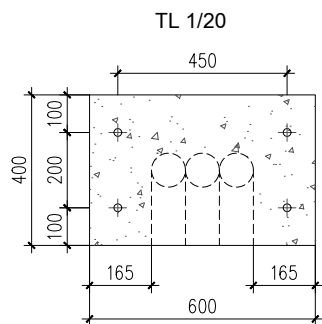
MẶT CẮT 1 - 1
