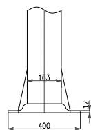
CHI TIẾT CHÂN CỘT ĐÈN
