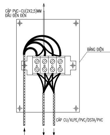
PHƯƠNG THỨC ĐẦU NỐI TẠI CỘT RỄ NHÁNH
