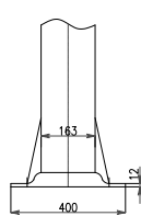
CHI TIẾT CHÂN CỘT ĐÈN
