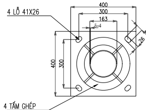
KHUNG MÓNG CỘT ĐÈN CHIẾU SÁNG 4XM24-300X300MM
